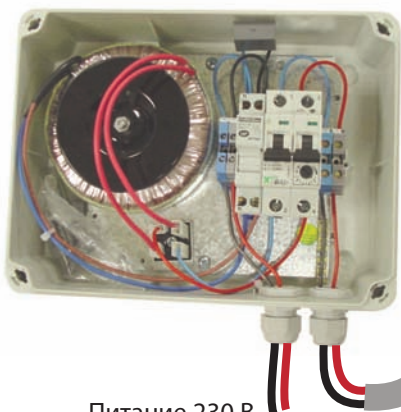
Питание 230 В
