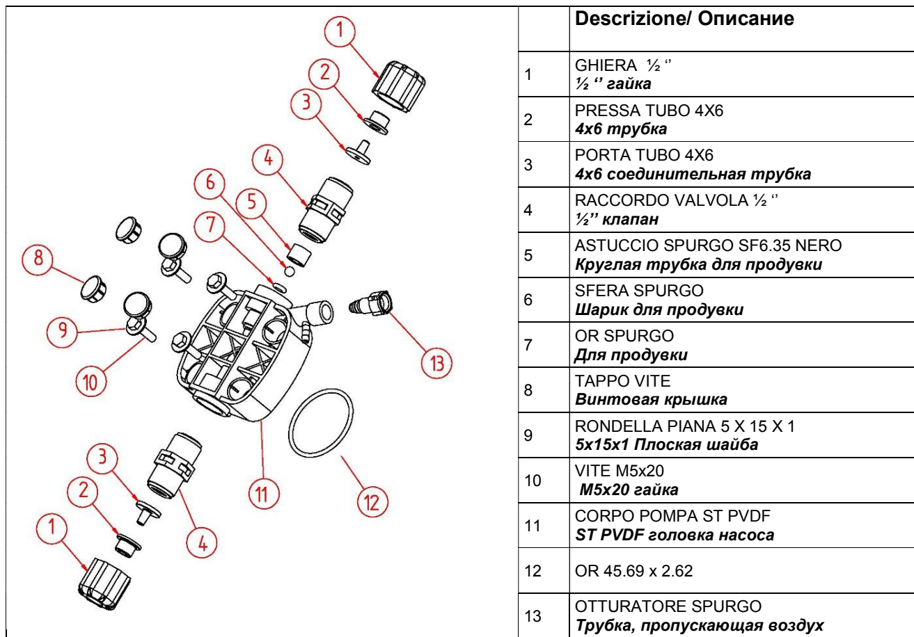
Fig. 1: Corpo pompa / Головка насоса
