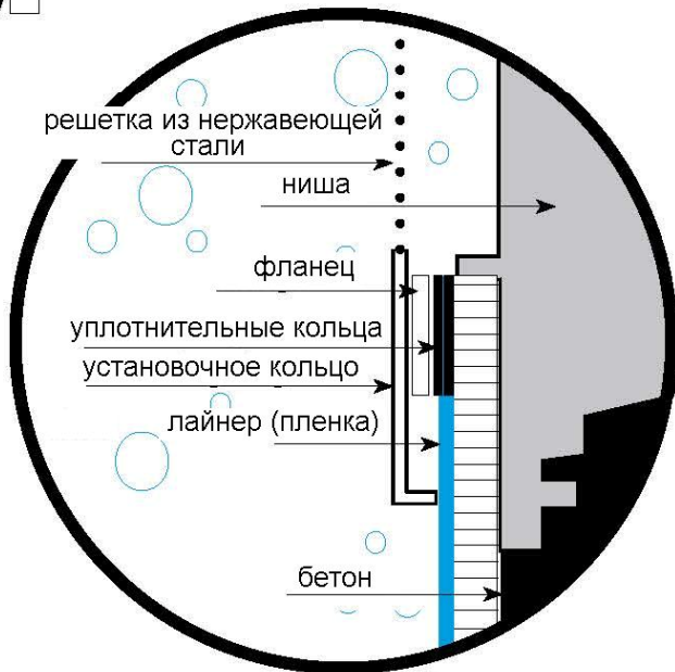
Пленочный бассейн
