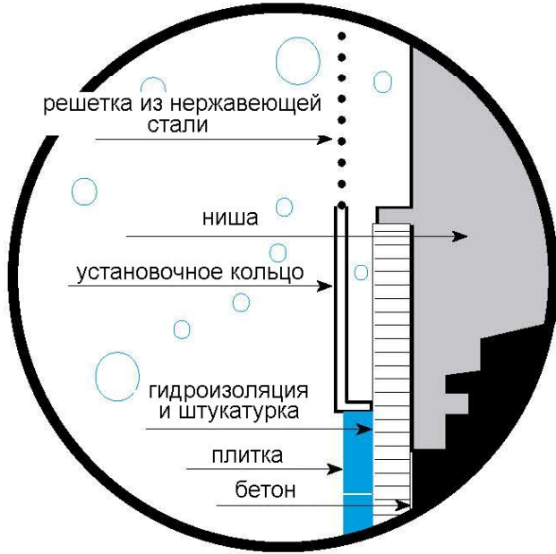
Бетонный бассейн
